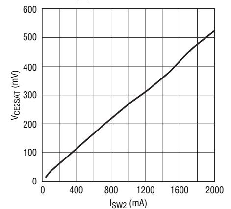
SW2 V_{\text{CESAT}}
