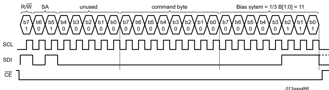
Fig 28. SPI-bus example
