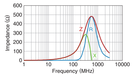
MMZ1608D800BTA00
