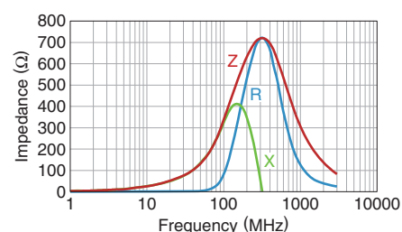
MMZ1608Q331BTA00
