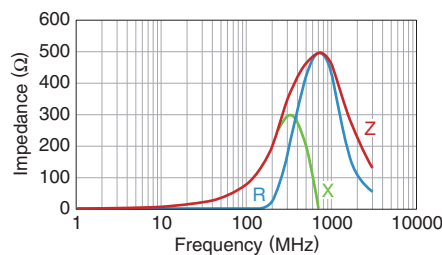
MMZ1608D800CTAH0
