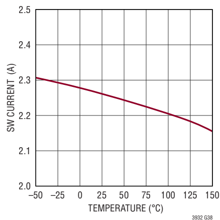
DA Current Limit
