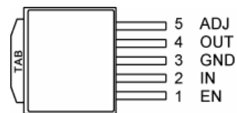
MIC39152WD TO-252-5 (D-Pak) (D)
