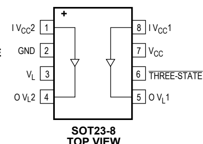
MAX3376E
