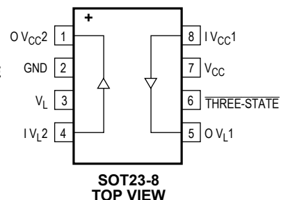
MAX3375E
