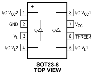
MAX3372E MAX3373E
