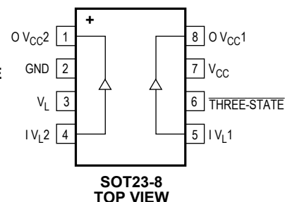
MAX3374E
