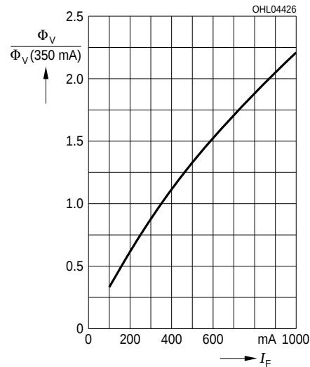
Relative Lichtstrom 2) Seite 21 Relative Luminous Flux 2) page 21 \Phi_V/\Phi_V(350\text{ mA}) = f(I_F); T_S = 25\text{ °C}
