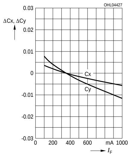
Farbortverschiebung 2) Seite 21 Chromaticity Coordinate Shift 2) Seite 21 x, y = f(I_F); T_S = 25\text{ °C}
