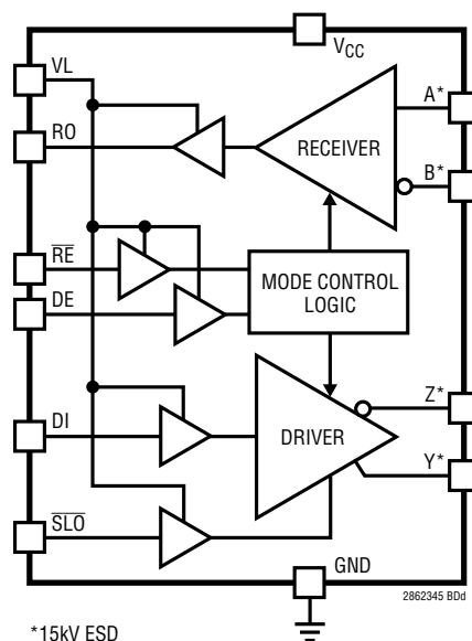
LTC2865
