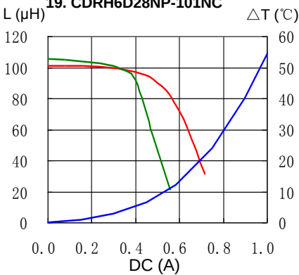
19. CDRH6D28NP-101NC
