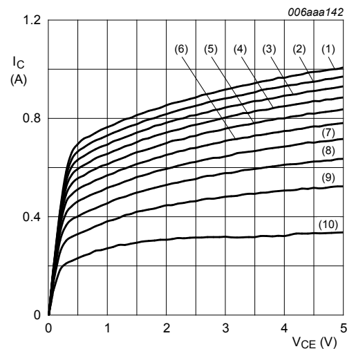
T_{amb} = 25\text{ }^{\circ}\text{C} (1) I_B = 12.0\text{ mA} (2) I_B = 10.8\text{ mA} (3) I_B = 9.6\text{ mA} (4) I_B = 8.4\text{ mA} (5) I_B = 7.2\text{ mA} (6) I_B = 6.0\text{ mA} (7) I_B = 4.8\text{ mA} (8) I_B = 3.6\text{ mA} (9) I_B = 2.4\text{ mA} (10) I_B = 1.2\text{ mA}
