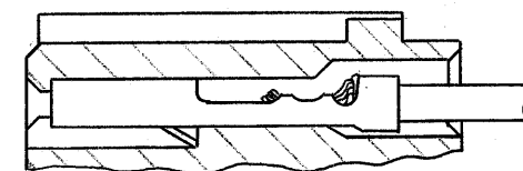
ファステーンファストン嵌合状態 (FASTIN-FASTON MATING STATE)
