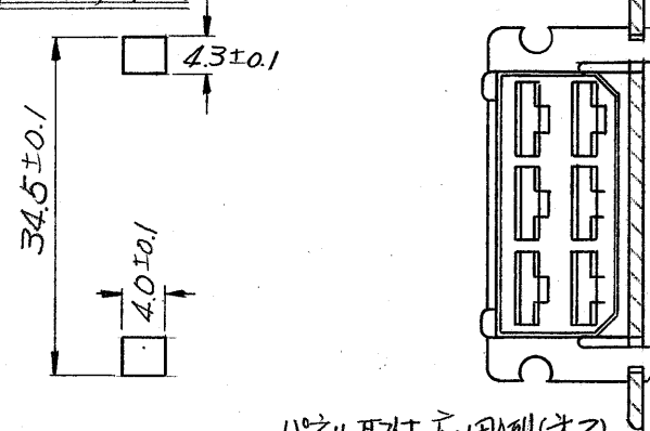
PANEL CUTTING DIMENSION パネル打抜寸法
