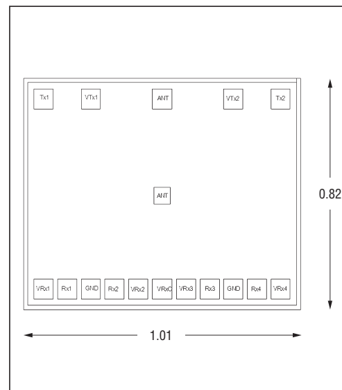
Die Layout
