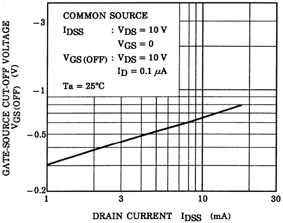
V_{GS}(\text{OFF}) - I_{DSS}
