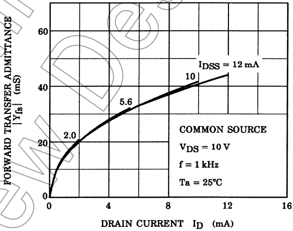
|Y_{fs}| - I_D
