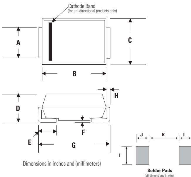
DO-214AB (SMC J-Bend)
