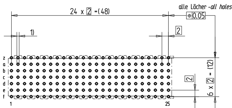
Lochbild für Leiterplatte (Bestückungsseite)
