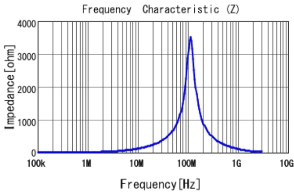
1231AS-H-2R2M |Z|
