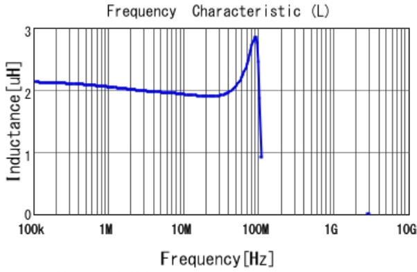
1231AS-H-2R2M L
