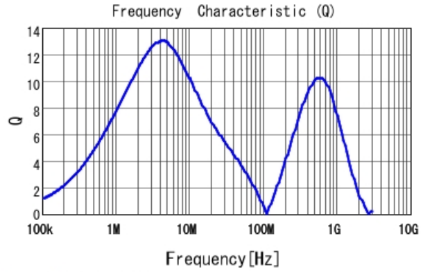
1231AS-H-2R2M Q
