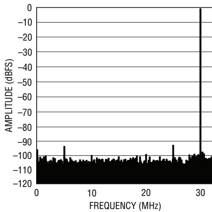
LTC2258-14: 8k Point FFT, f_{IN} = 30\text{MHz} , -1\text{dBFS} , 65\text{Msps}
