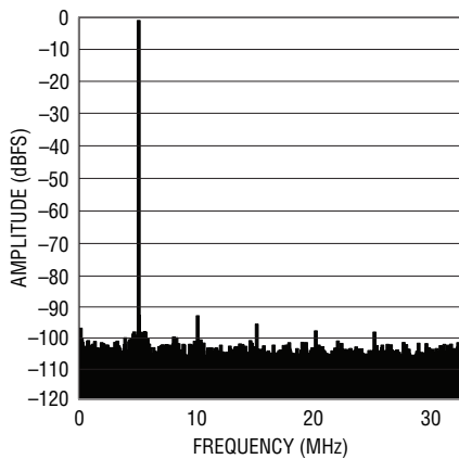
LTC2258-14: 8k Point FFT, f_{IN} = 70\text{MHz} , -1\text{dBFS} , 65\text{Msps}
