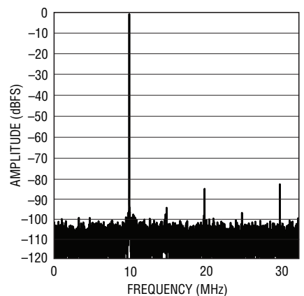
LTC2258-14: 8k Point FFT, f_{IN} = 140\text{MHz} , -1\text{dBFS} , 65\text{Msps}
