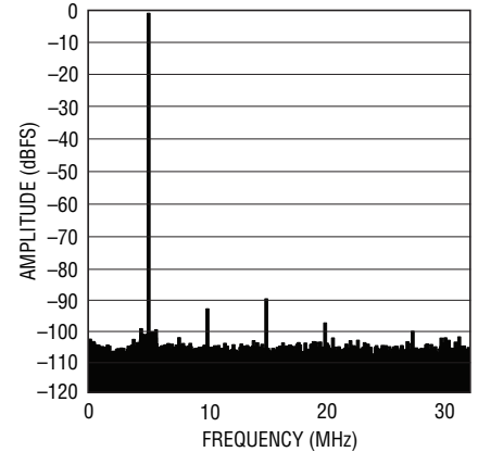
LTC2258-14: 8k Point FFT, f_{IN} = 5\text{MHz} , -1\text{dBFS} , 65\text{Msps}
