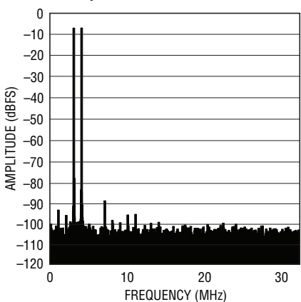
LTC2258-14: 8k Point 2-Tone FFT, f_{IN} = 68\text{MHz} , 69\text{MHz} , -1\text{dBFS} , 65\text{Msps}
