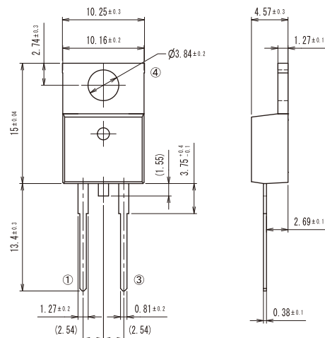
<A-16> TO-220
