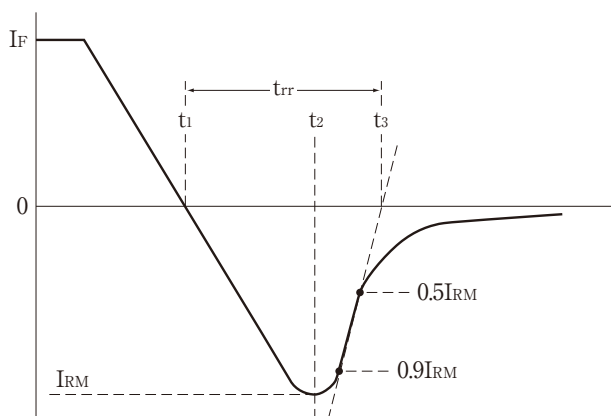
図 1. 逆回復波形
