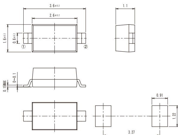
<A-5> SOD-123
