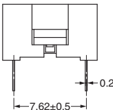
Flat Actuator
