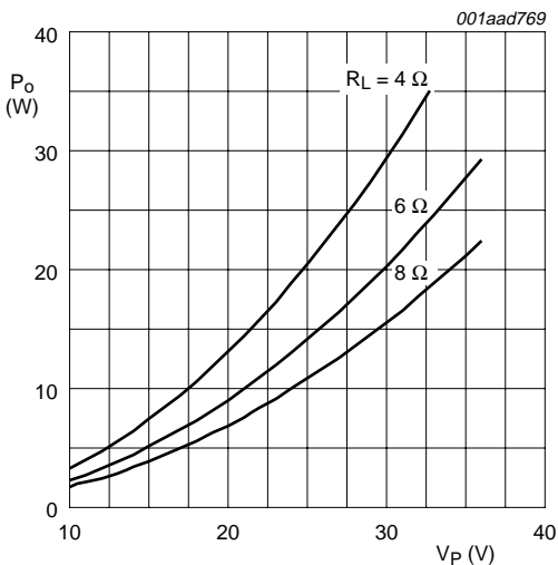
b. THD+N = 10 %
