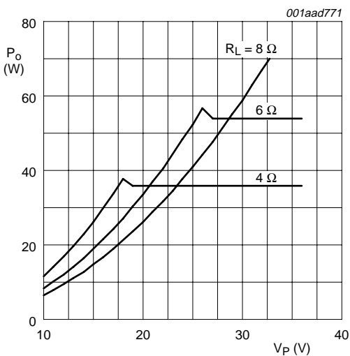
b. THD+N = 10 %
