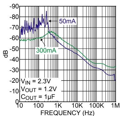
PSRR
