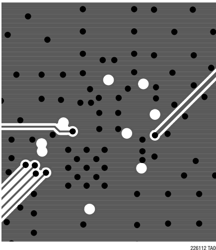
Inner Layer 3
