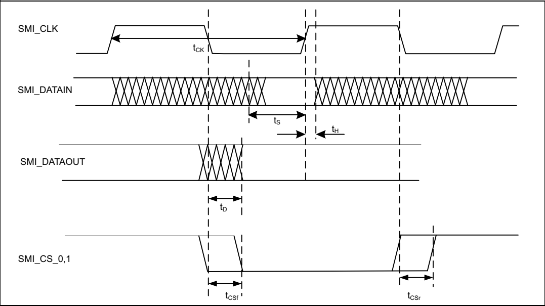
Figure 30. SMI input/output waveform
