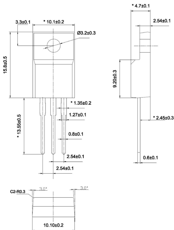
ITO-220-AB
