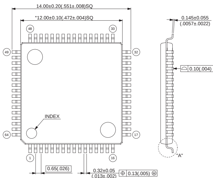
64-pin plastic LQFP (FPT-64P-M23)
