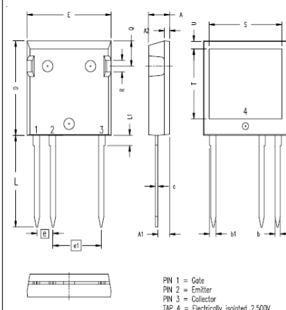
ISOPLUS i4-Pak™ (HV) (IXGF) Outline
