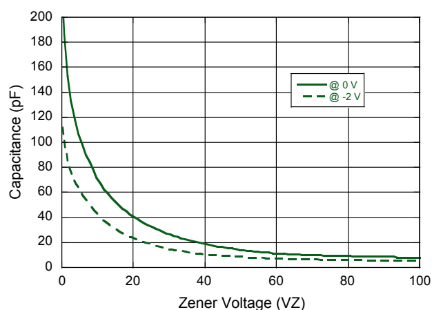
Capacitance vs. Zener Voltage
