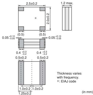
CSACW_X 20.01-70.00MHz
