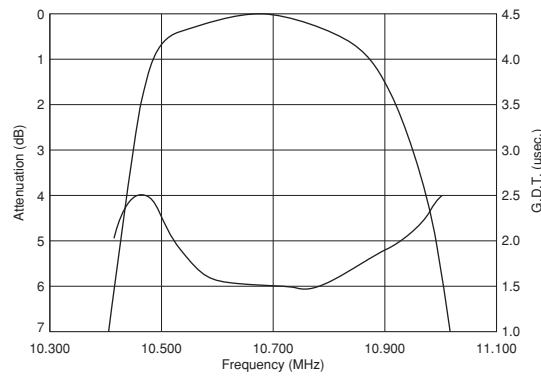
SFELF10M7DF00-B0
