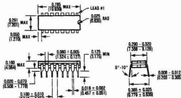
16 Lead Cerdip (JE)
