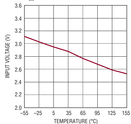
V_{IN} UVLO
