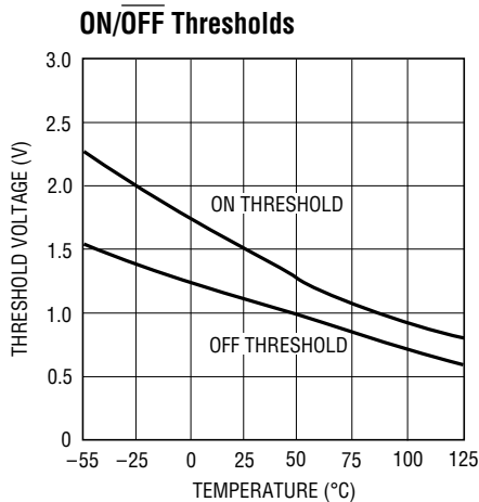
LT1342 • TPC07
