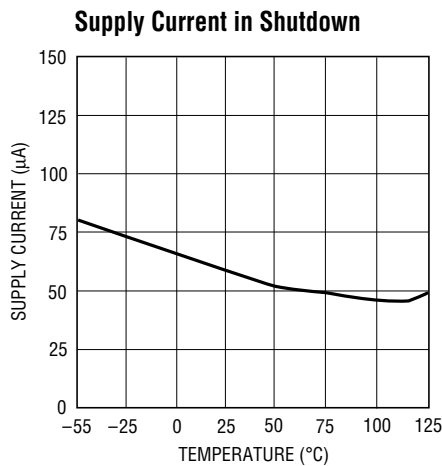
LT1342 • TPC04
