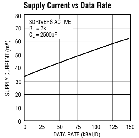
LT1342 • TPC03
