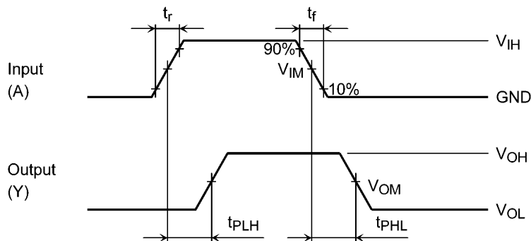
Fig. 11.6.1 t_{PLH} , t_{PHL}
