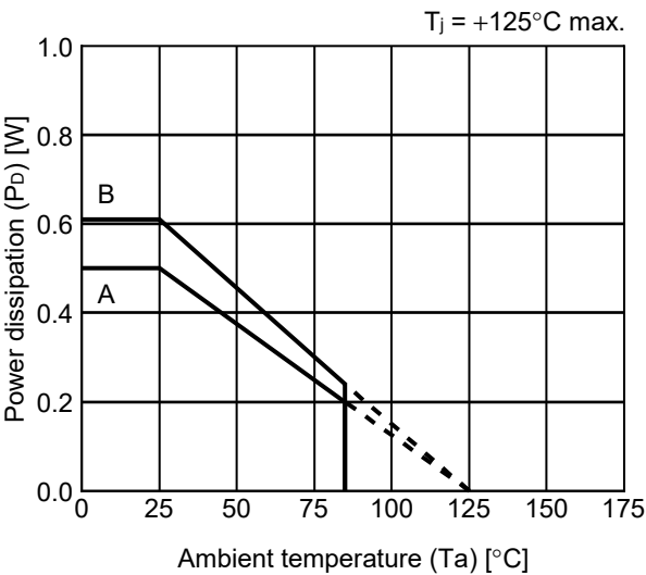
SOT-23-3
