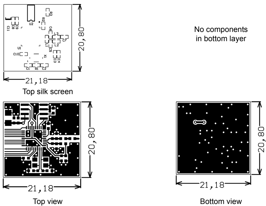
Figure 28. nRF24Z1 ARX PCB layout
