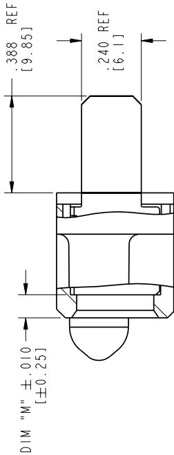
SECTION B-B SCALE 2:1
