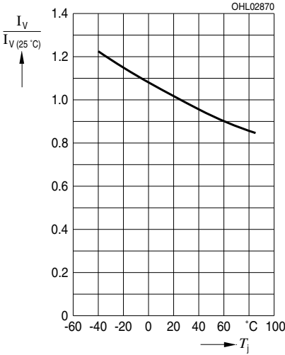
Relative Luminous Intensity 7) page 20 Relative Lichtstärke 7) Seite 20 I_V/I_V(25^\circ\text{C}) = f(T_j); I_F = 30\text{ mA}
