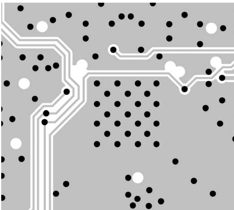
Inner Layer 3
