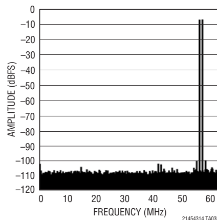
64k Point 2-Tone FFT, f_{IN} = 69\text{MHz} , 70\text{MHz} , -1\text{dBFS} , 125\text{Mps}
