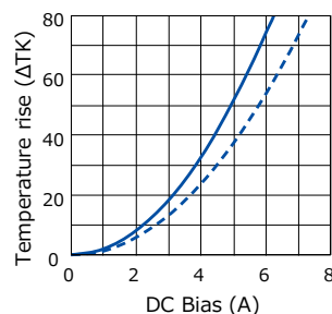
[ ETQP4M100KVK ]
