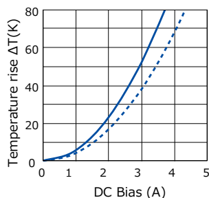
[ ETQP4M330KVK ]
