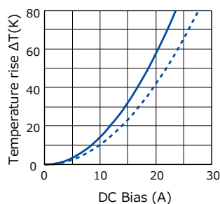
[ ETQP4MR68KVK ]
