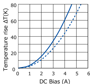
[ ETQP4M220KVK ]
