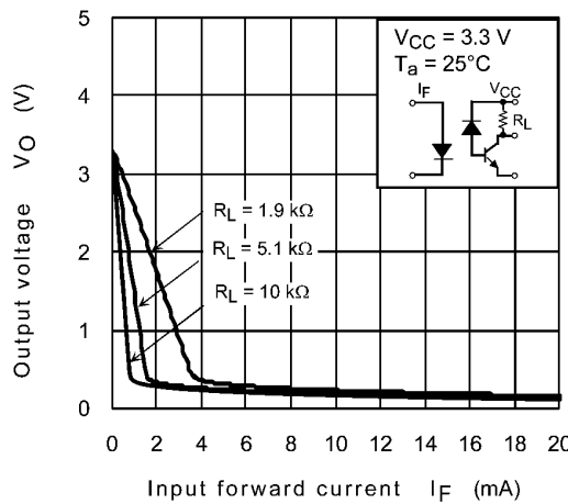
Fig. 12.2.14 V_O - I_F
