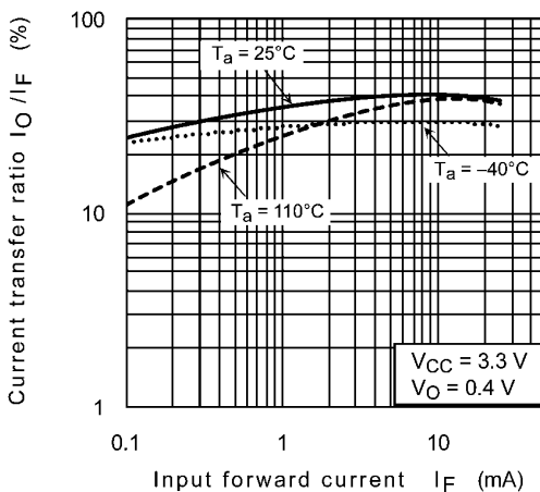
Fig. 12.2.6 I_O/I_F - I_F
