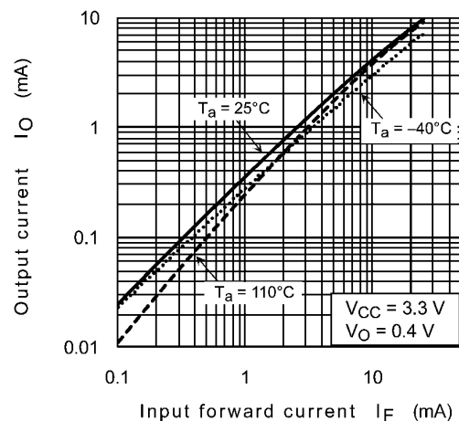
Fig. 12.2.5 I_O - I_F
