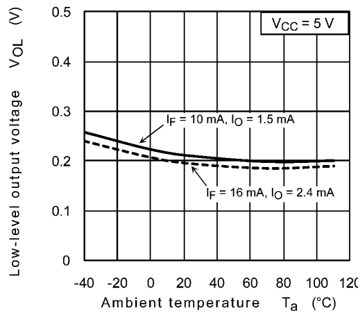
Fig. 12.2.15 V_{OL} - T_a
