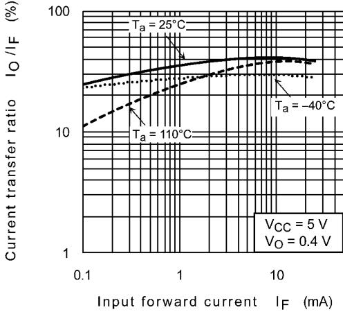
Fig. 12.2.4 I_O/I_F - I_F
