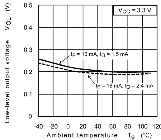
Fig. 12.2.16 V_{OL} - T_a
