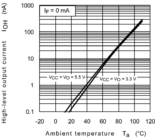
Fig. 12.2.2 I_{OH} - T_a
