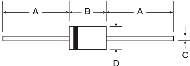
DO-201AD
