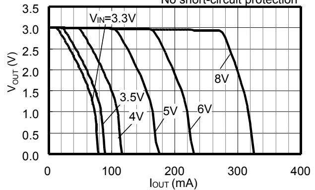
S-812C30A (Ta=25°C)
