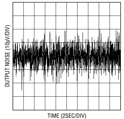
5V Output Noise 0.1\text{Hz} \leq f \leq 10\text{Hz}
