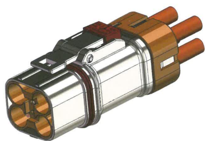
4芯插头 4POS Plug
