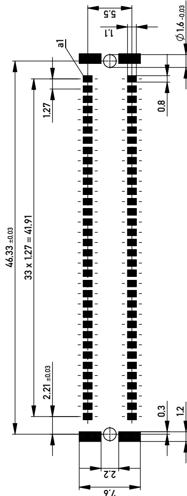
Leiterplatten-Layout Vorschlag für SMT PCB-Layout Proposal for SMT
