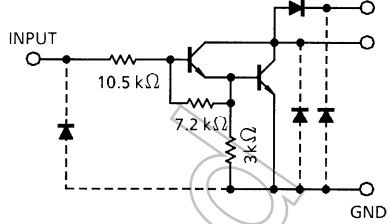
ULN2804APG / AFWG
