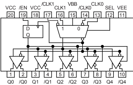
20-Pin TSSOP
