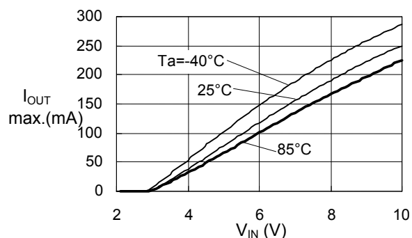
S-817B30A
