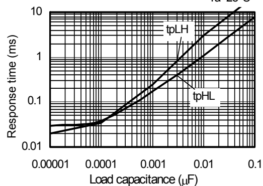
S-80960CN T_a=25^\circ\text{C}
