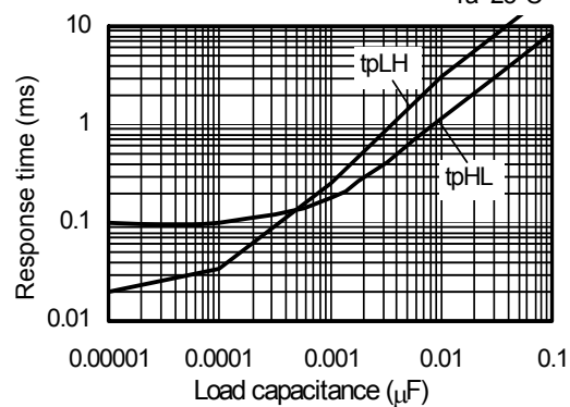
S-80960CN T_a=25^\circ\text{C}
