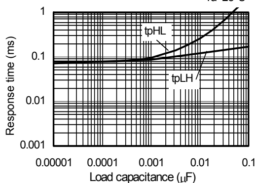
S-80960CL T_a=25^\circ\text{C}
