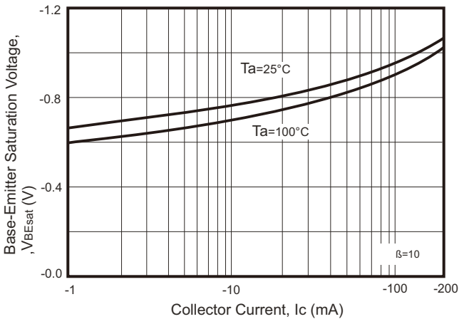
Fig. 4 - V_{BEsat} - I_c
